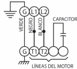
MONOFÁSICO 115V CA CABLE DE ALIMENTACIÓN 3x14
