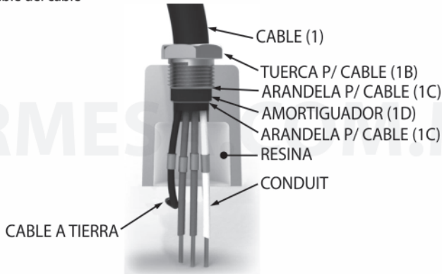
Figura 2: Ensamble del cable
