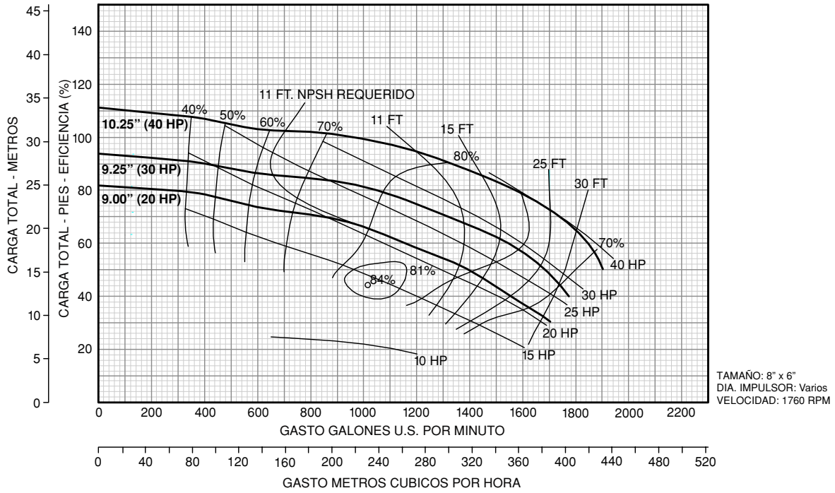
Modelo HC-8x6-10
